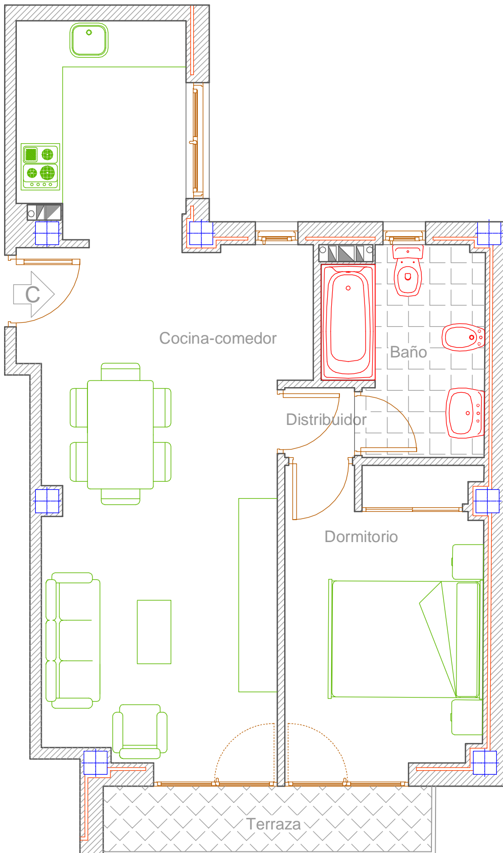
APARTAMENTO TIPO C Superficie: 52.58 m 2
